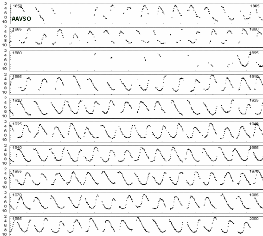
Рис. 14. Кривая изменения блеска классической долгопериодической переменной звезды – Миры Кита за период с 1850 по 2000г с 10-дневным интервалом между наблюдениями. ( www.aavso.org ) Средний интервал изменения блеска Миры - 3,5-9m. Период изменения блеска - 332 дня.
