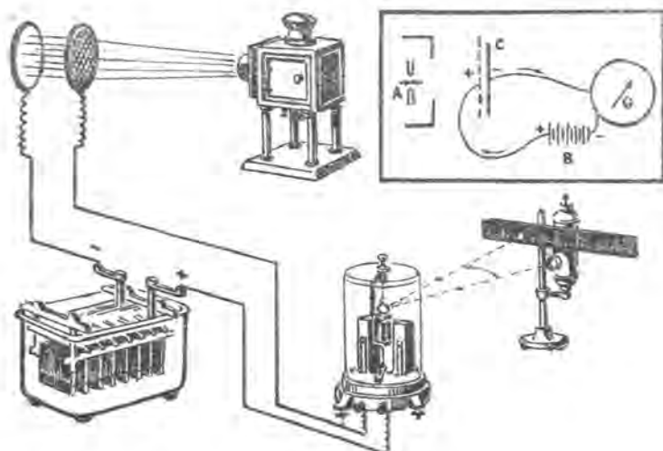
Схема опыта Столетова по исследованию актиноэлектрических явлений. В рамке — рисунок из сочинения Столетова.
