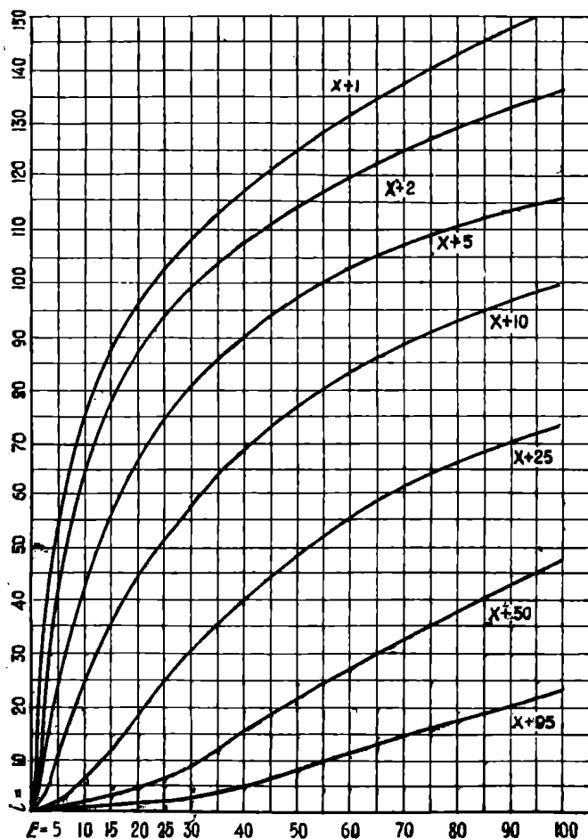
Кривые, снятые Столетовым, показывающие зависимость силы фототока от величины электрического напряжения.
