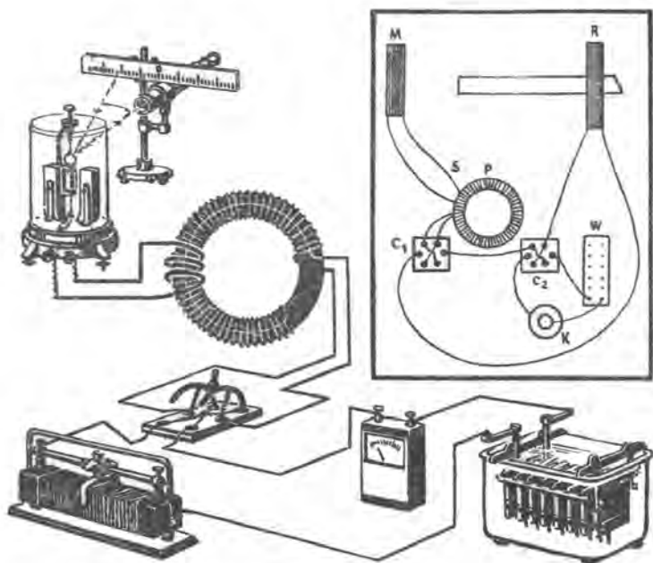
Схема опыта Столетова по исследованию магнитных свойств железа. В рамке — рисунок из сочинения Столетова.
