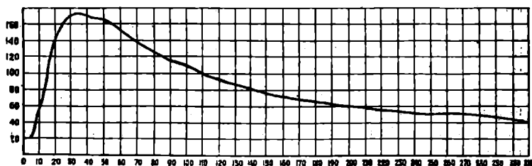
Кривая, снятая Столетовым, показывающая зависимость магнитной восприимчивости от величины намагничивающего поля.
