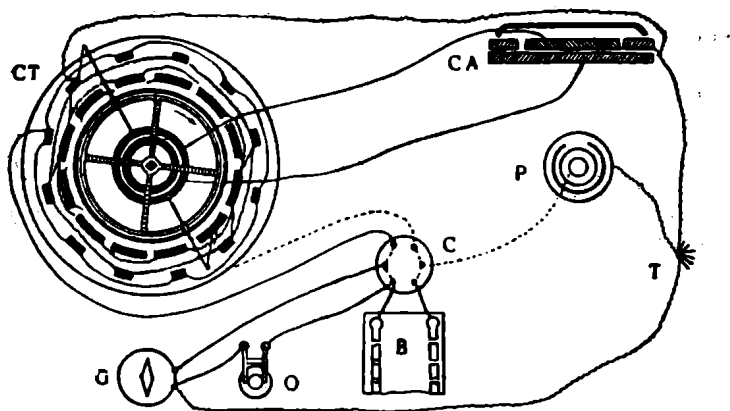
Схема установки Столетова для определения скорости электромагнитных процессов.
