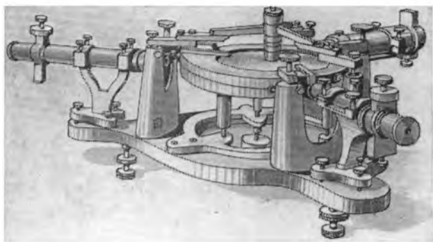
Конденсатор Столетова.
